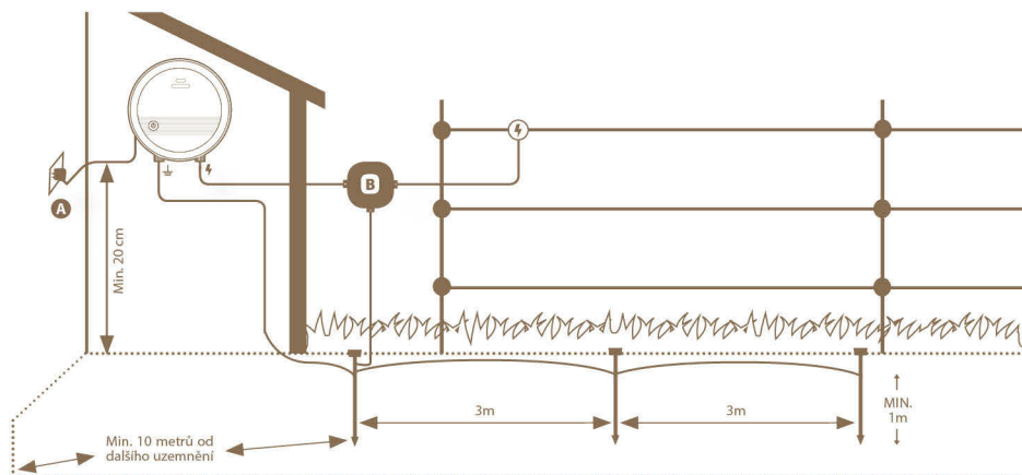
Obrázek č. 3: Montáž generátoru a uzemnění
