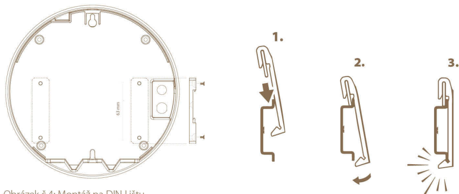
Obrázek č.4: Montáž na DIN Lištu
